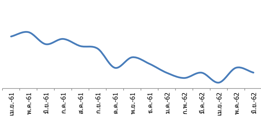
ปริมาณการใช้แท่งถ่านอิเล็กโทรด เตาลหอม (กิโลกรัม/ตัน)-SISCO
